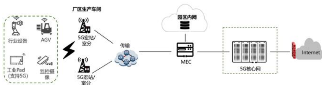
图 4-4 园区 5G 专网部署
