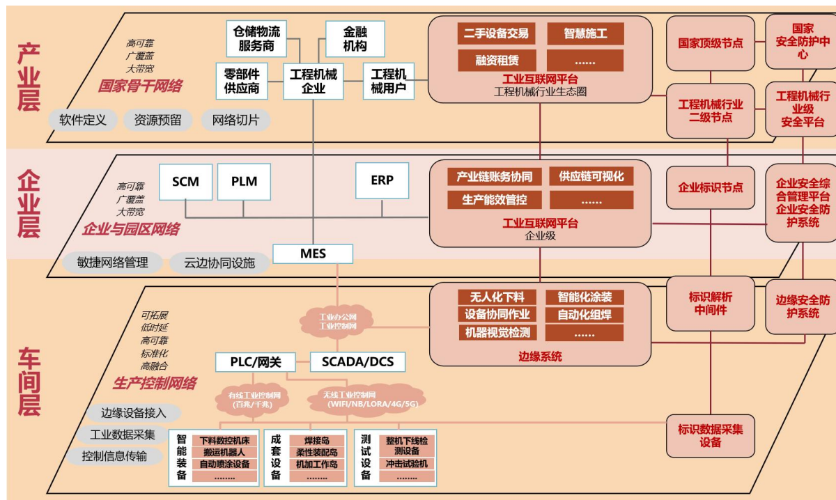
图 3-2 工程机械行业工业互联网融合创新实施架构 8
